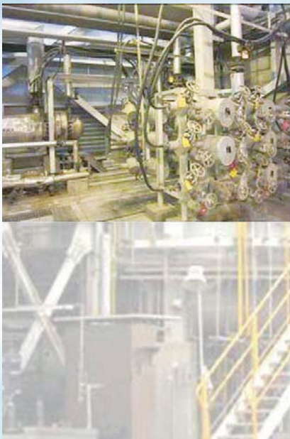
製程蒸汽進口閥XPV-151， 改為DCS控制， 提升膨脹機XC-151發電量。
