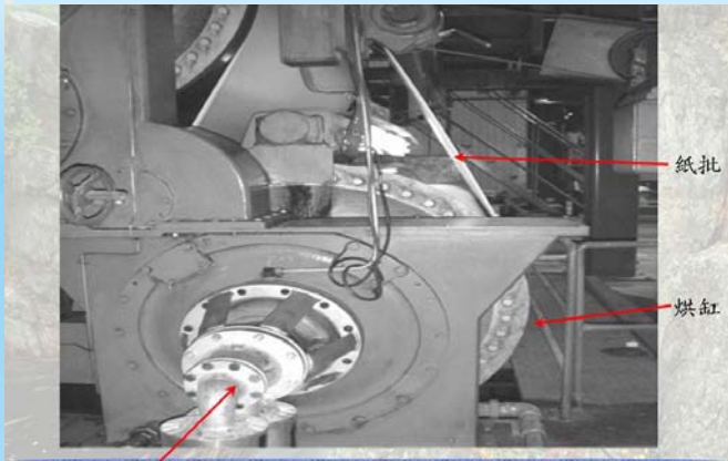
乾燥紙張之烘缸中清除積水之虹吸管由原迴轉式汰換為效能較高之固定式虹吸管，降低蒸氣用量。
